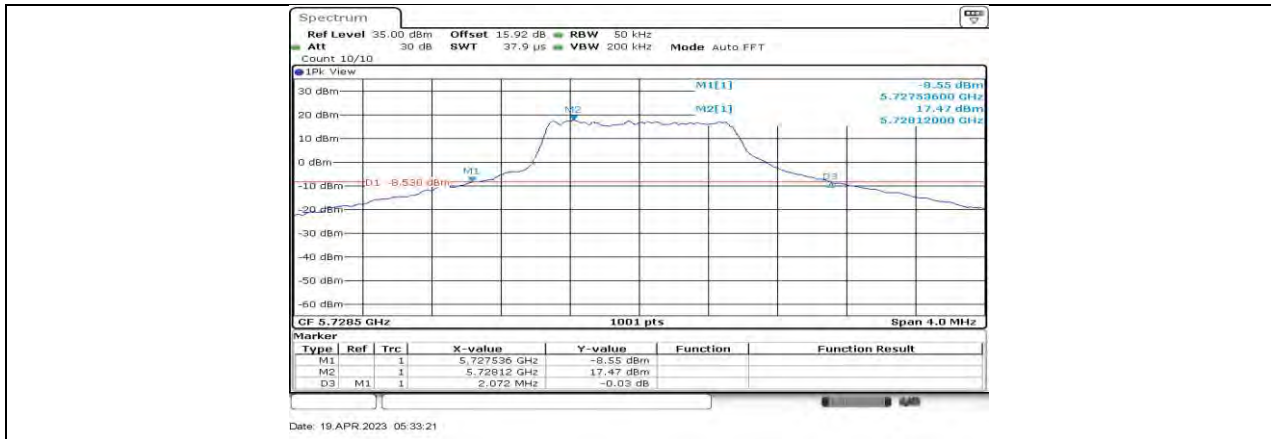
1.4 MHz Ant1 5728.5
