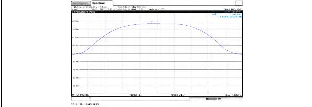
1.4 MHz_Ant0_5846.5
