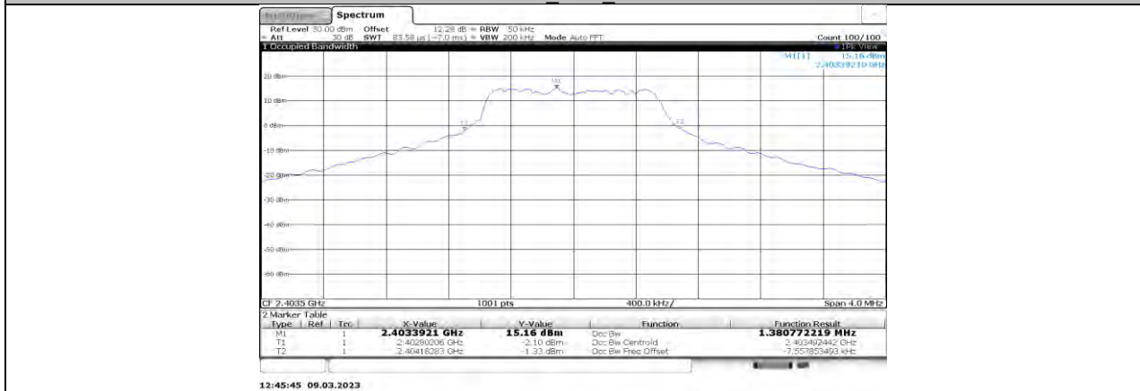
1.4 MHz_Ant1_2403.5
