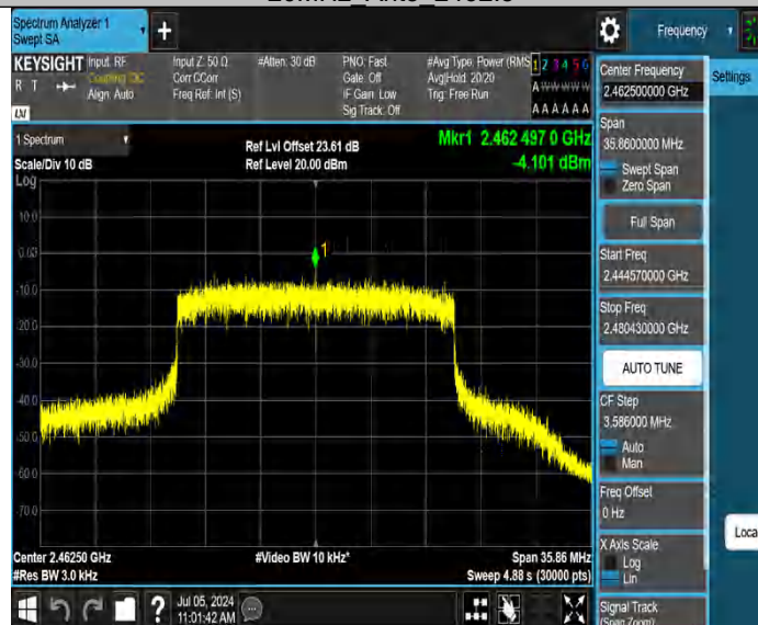
20MHz Ant6 2462.5
