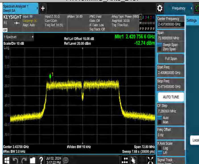
11N40MIMO Ant0 2437
