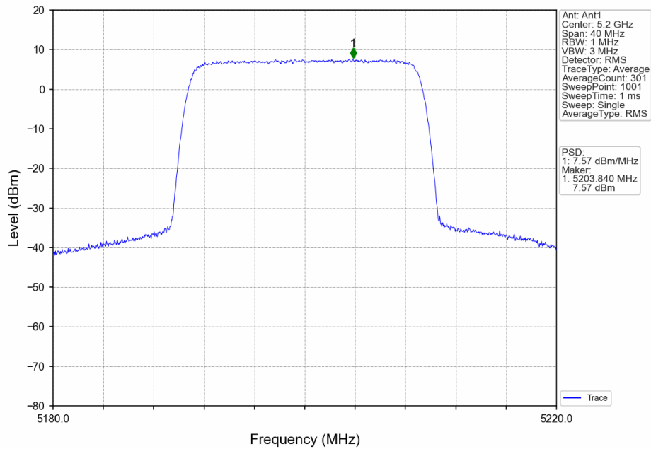
20_MCH_5200MHz_Ant1_NTNV
