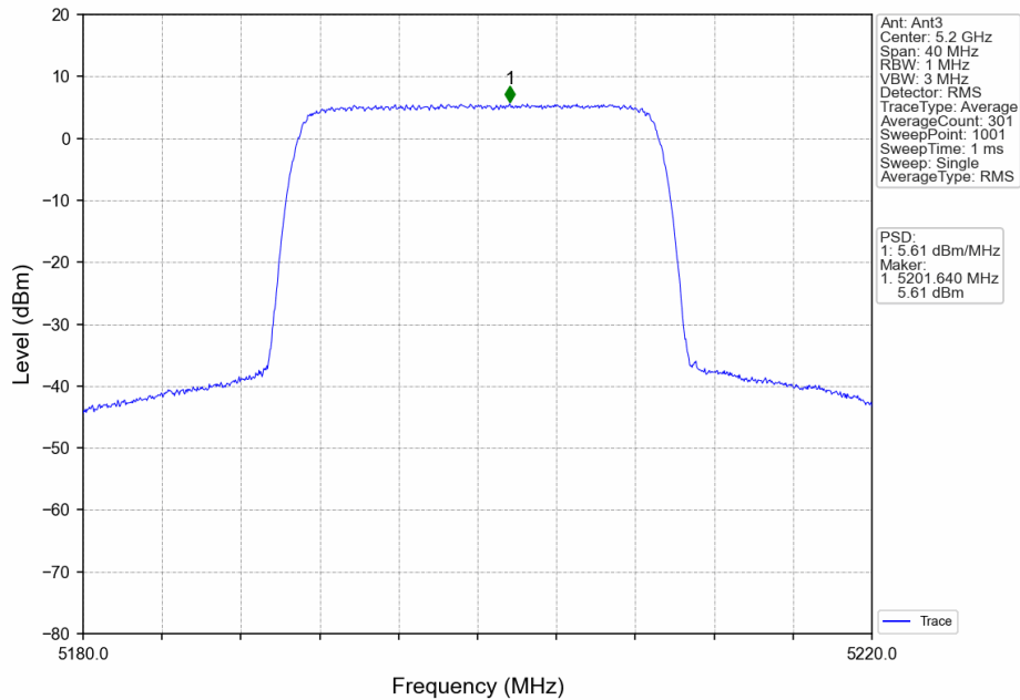
20_MCH_5200MHz_Ant3_NTNV
