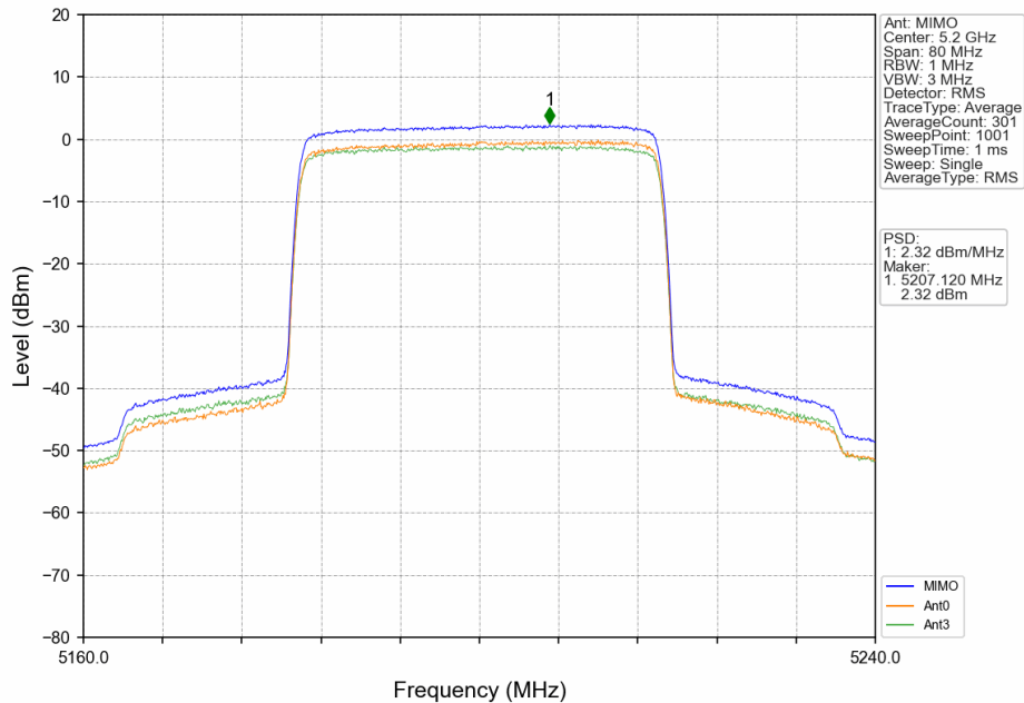
40_MCH_5200MHz_MIMO_NTNV
