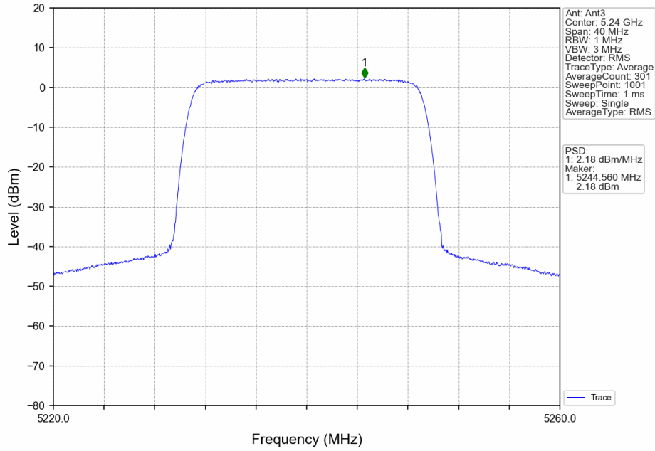
20_HCH_5240MHz_MIMO_NTNV
