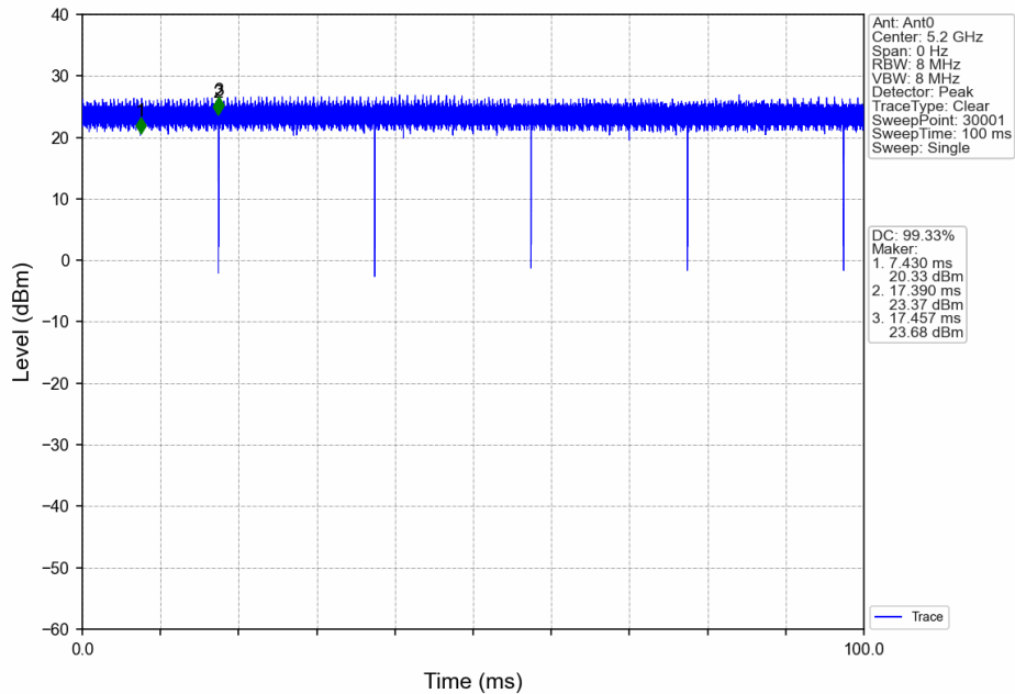
40_MCH_5200MHz_Ant0_NTNV
