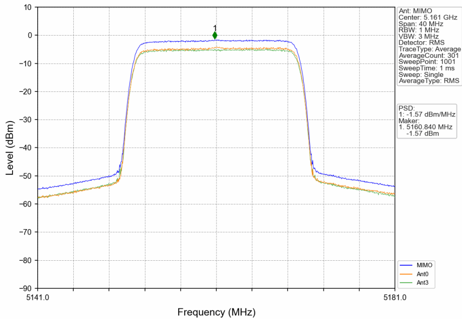
20_LCH_5161MHz_MIMO_NTNV
