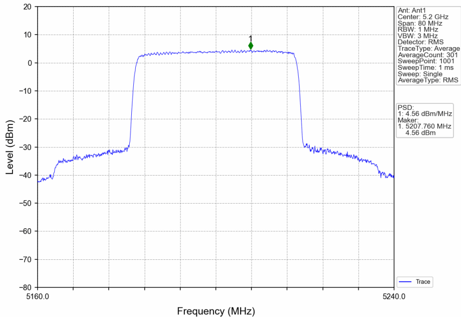
40_MCH_5200MHz_Ant1_NTNV
