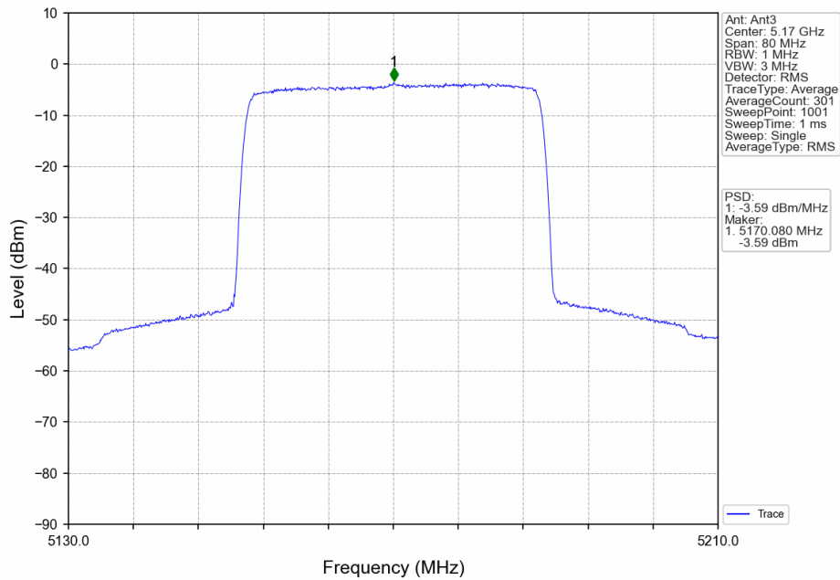
40_LCH_5170MHz_Ant3_NTNV
