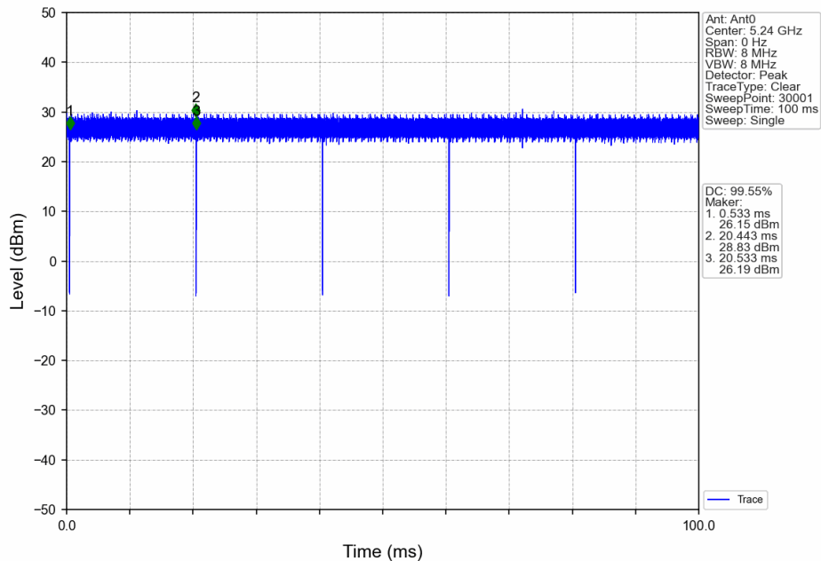
20_HCH_5240MHz_Ant0_NTNV
