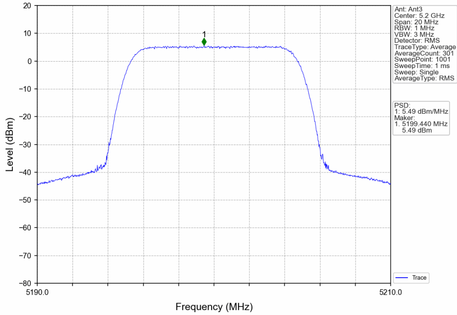
10_MCH_5200MHz_MIMO_NTNV
