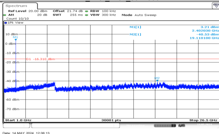
LE 2M Ant1 2402 1000~26500
