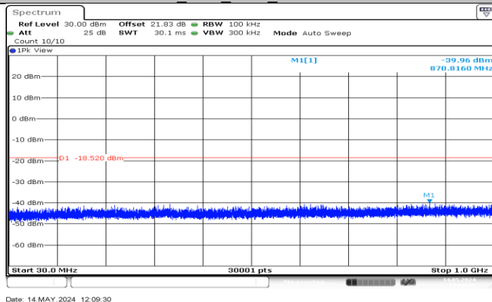
LE 2M Ant1 2440 0~Reference
