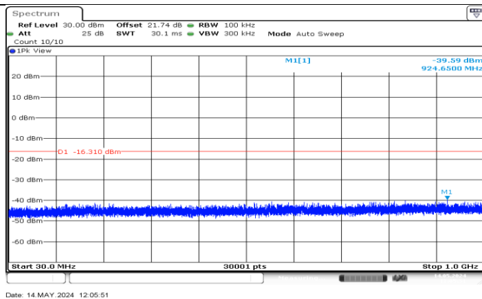
LE 2M Ant1 2402 30~1000
