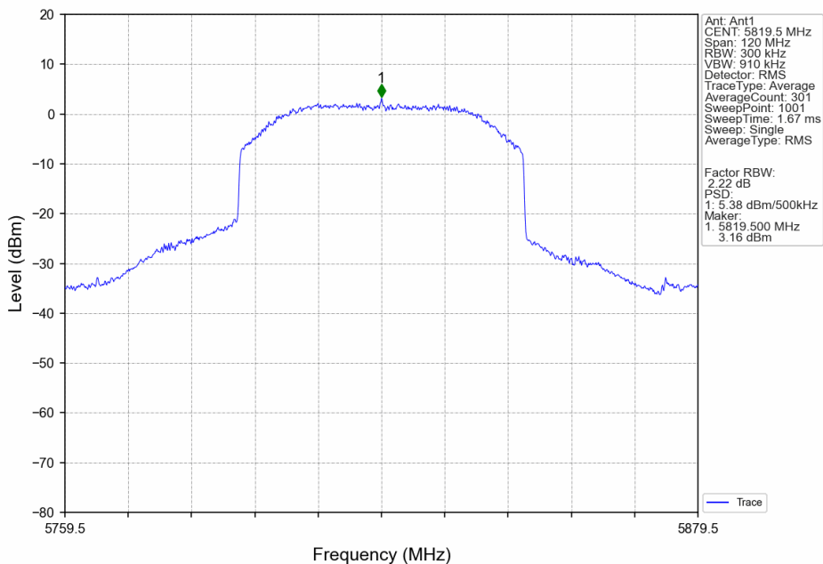
60M_HCH_5819.5MHz_MIMO_NTNV
