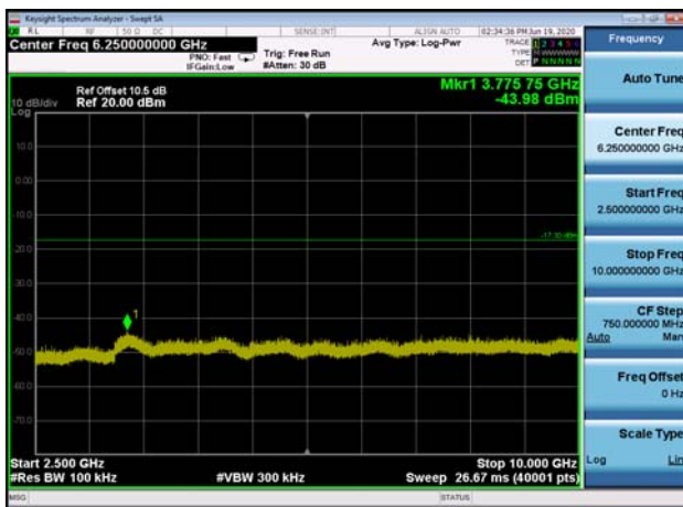
,Plot 4,2500MHz~10000MHz-802.11g ,2462MHz
