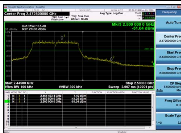
,Plot 2,Band Edge-802.11n(HT20) ,2462MHz
