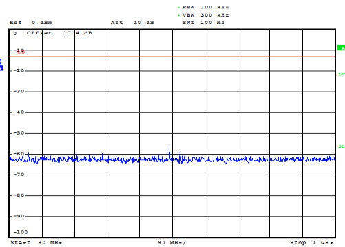
GSM 1900 CH-Middle 30MHz~1GHz
