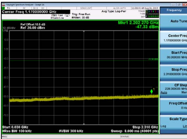
,Plot 3,30MHz~2310MHz-802.11b,2462MHz
