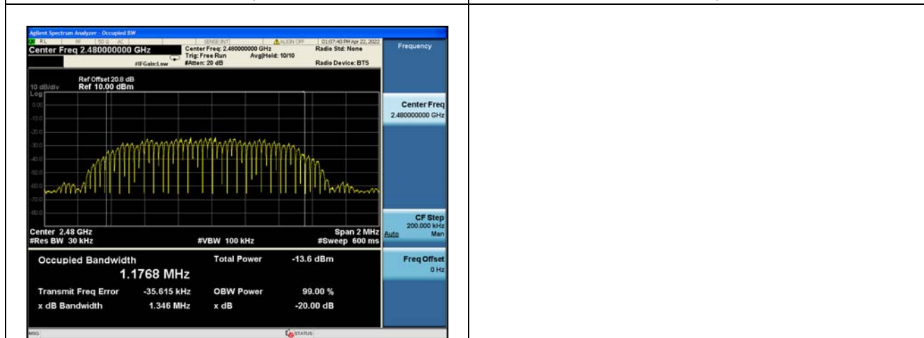
Modulation: \pi/4 DQPSK 2480MHz
