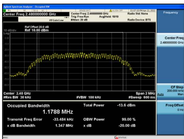
Modulation: \pi/4 DQPSK 2480MHz
