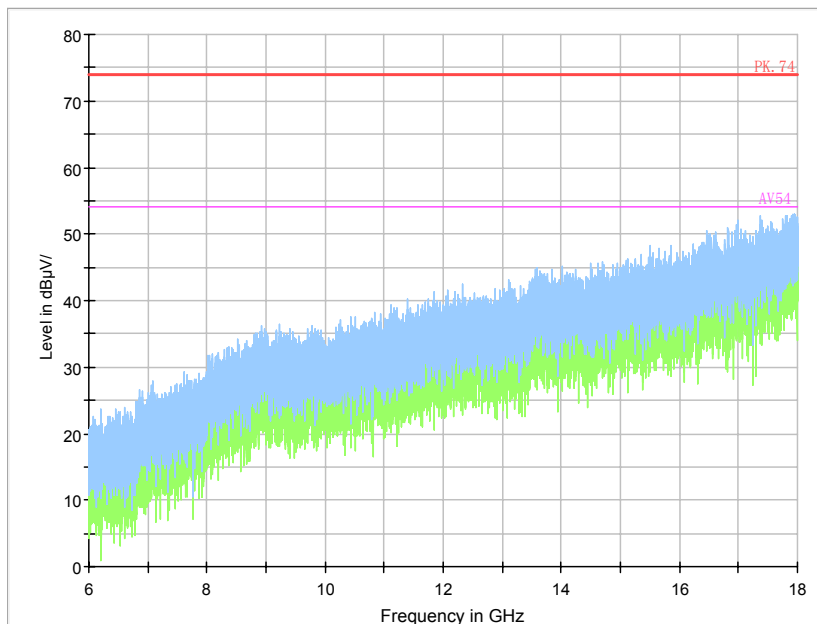
Frequency Range: 6GHz - 18GHz Detector: Av mode and PK mode Modulation type: 802.11ac MIMO (VHT80)
