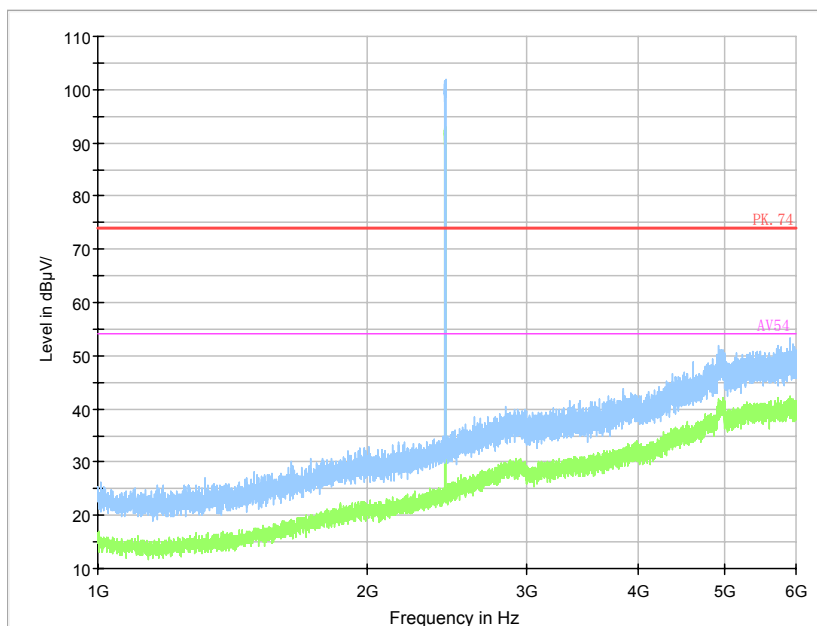
Frequency Range: 1GHz - 6GHz Detector: Av mode and PK mode Modulation type: 802.11ac MIMO (VHT80)
