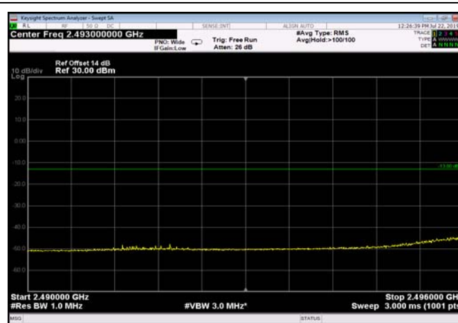
FDD07_5MHz_2502.5_Q16_OneRB_low _ExtraBands_Range_2490~2496
