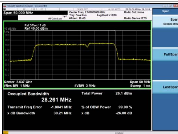
FDD7_MidRange_20+10_QPSK
