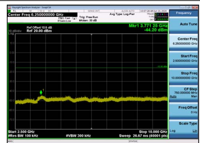
,Plot 4,2500MHz~10000MHz-802.11n(HT20),2462MHz,Ant1
