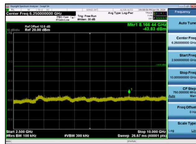
,Plot 4,2500MHz~10000MHz-802.11n(HT20),2437MHz,Ant0
