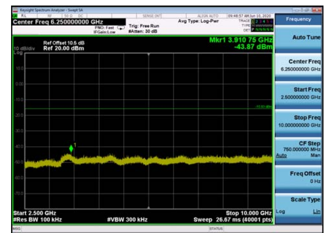
,Plot 4,2500MHz~10000MHz-802.11n(HT20),2437MHz,Ant1
