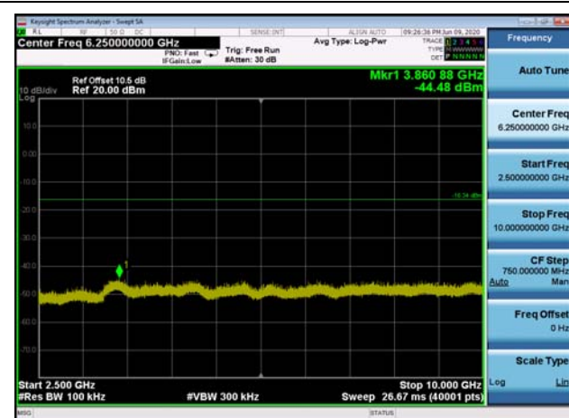
,Plot 4,2500MHz~10000MHz-802.11n(HT20),2462MHz,Ant0
