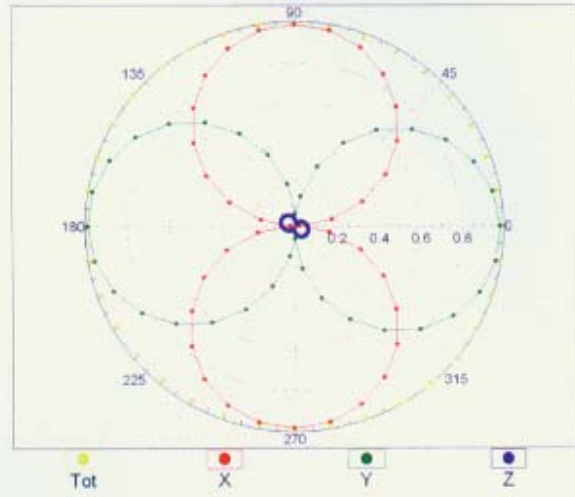
f=2500 MHz,R22,0°
