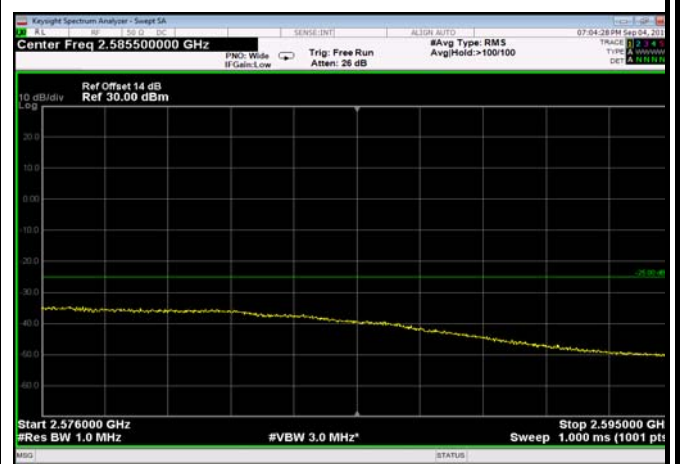
FDD07_20MHz_2560_QPSK_fullIRB_ExtraBan ds_Range_2576~2595
