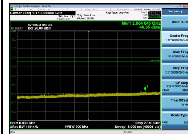
,Plot 3,30MHz~2310MHz-802.11g,2437MHz
