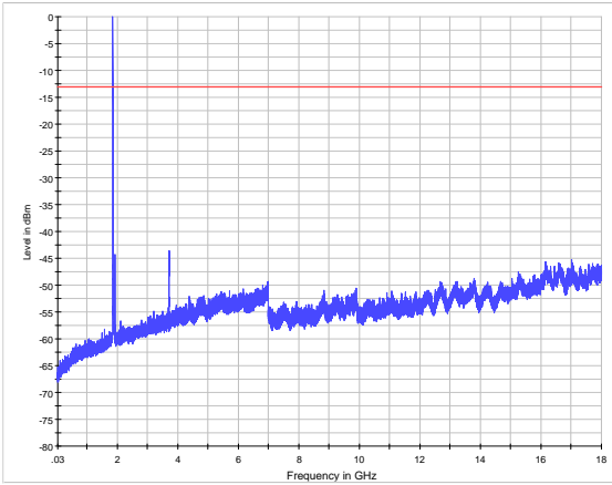
WCDMA Band II CH-Middle 30MHz~18GHz
