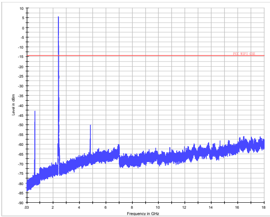
802.11b CH6 30MHz to 18GHz
