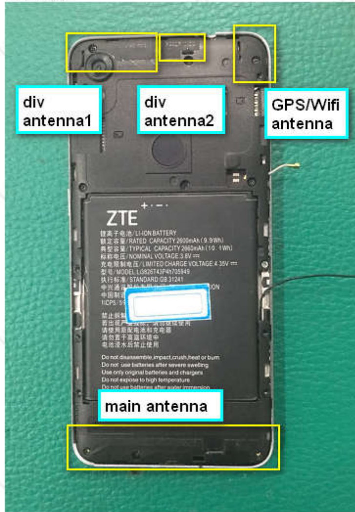
天线位置图
