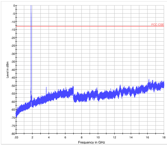
WCDMA Band II CH-Middle 30MHz~18GHz
