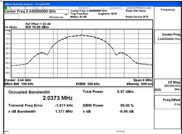
Test Mode:GFSK (LE 2Mbps)
