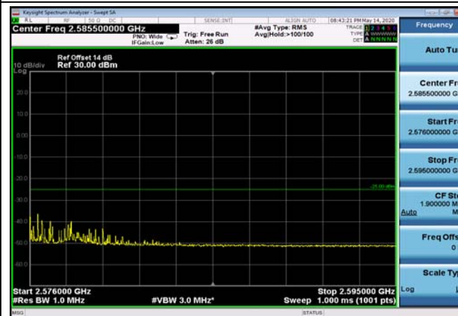
FDD07_5MHz_2567.5_Q16_OneRB_high _ExtraBands_Range_2576~2595
