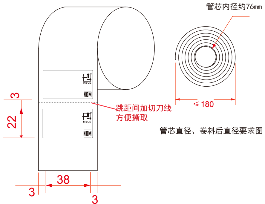
贴纸卷料方向图示
