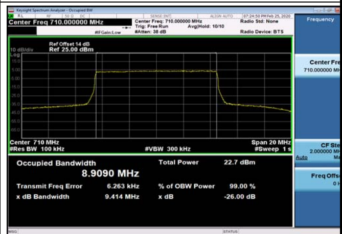
FDD17_MidRange_10_710_Q16
