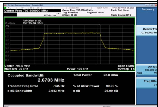
FDD12_MidRange_3_707.5_Q16
