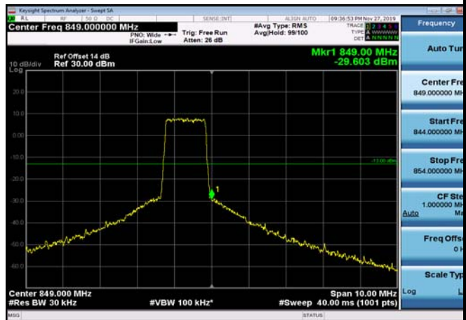
HighRange_FDD05_3MHz_847.5_OneRB_high_Q16
