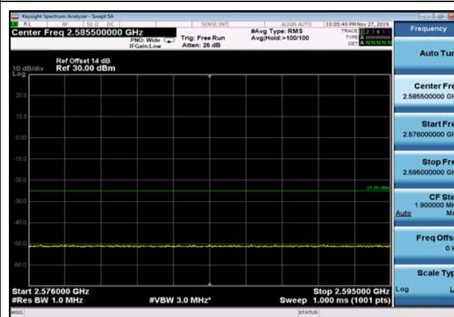
FDD07_20MHz_2510_Q16_fullIRB_ExtraBand s_Range_2576~2595
