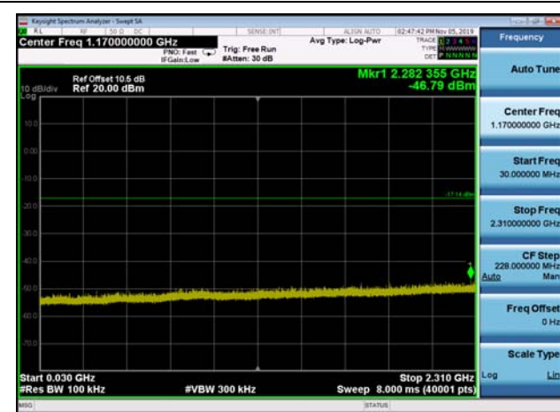
,Plot 3,30MHz~2310MHz-802.11g,2437MHz
