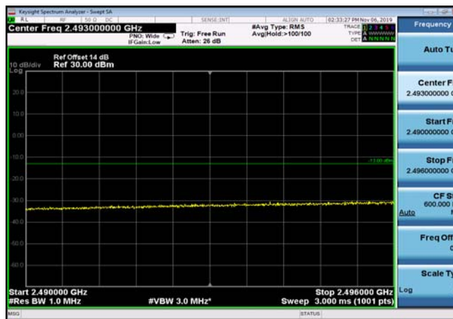
FDD07_20MHz_2510_Q16_fullRB_ExtraBand s_Range_2490~2496
