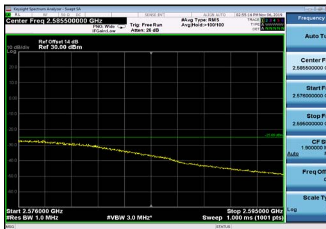
FDD07_20MHz_2560_QPSK_fullIRB_ExtraBan ds_Range_2576~2595
