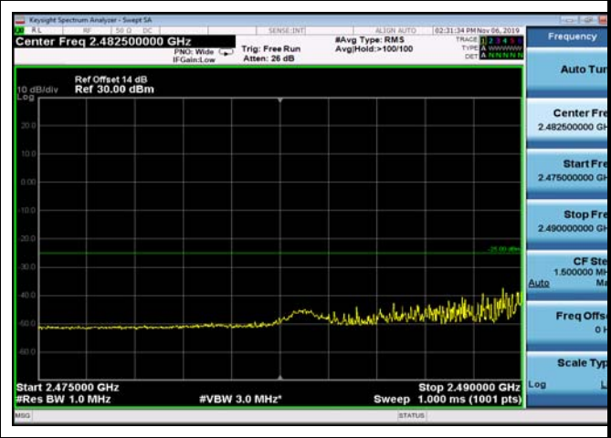
FDD07_20MHz_2510_Q16_OneRB_low _ExtraBands_Range_2475~2490
