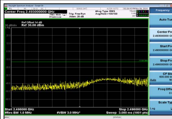
FDD07_15MHz_2507.5_Q16_OneRB_low _ExtraBands_Range_2490~2496
