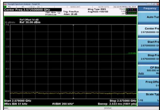
FDD07_20MHz_2510_Q16_fullRB_ExtraBand s_Range_2570~2575
