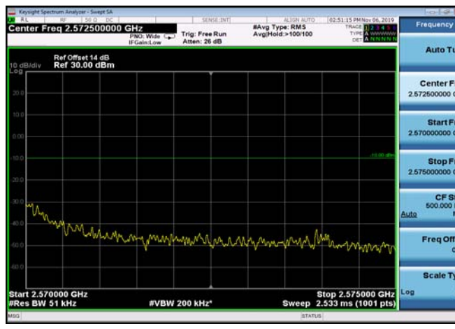
FDD07_20MHz_2560_Q16_OneRB_high _ExtraBands_Range_2570~2575
