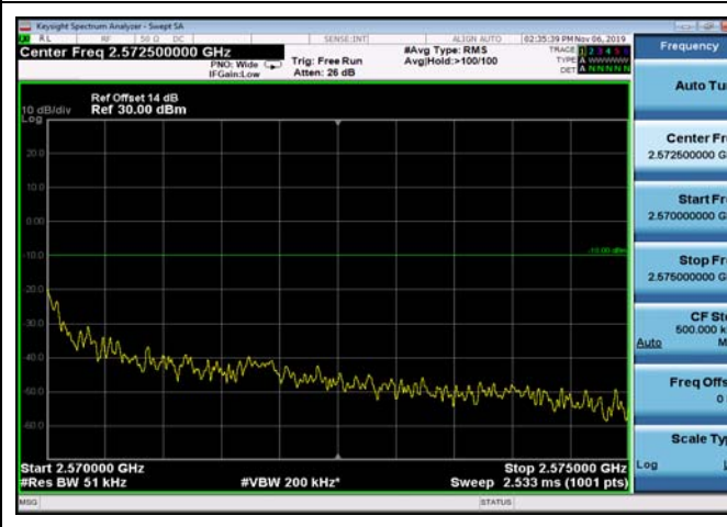
FDD07_5MHz_2567.5_Q16_OneRB_high _ExtraBands_Range_2570~2575
