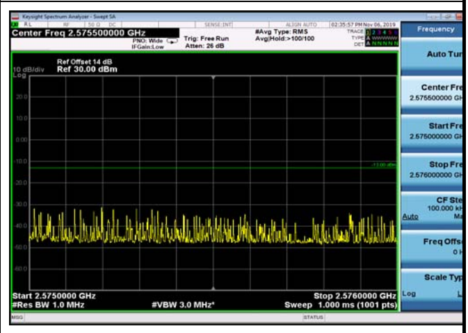
FDD07_5MHz_2567.5_Q16_OneRB_high _ExtraBands_Range_2575~2576
