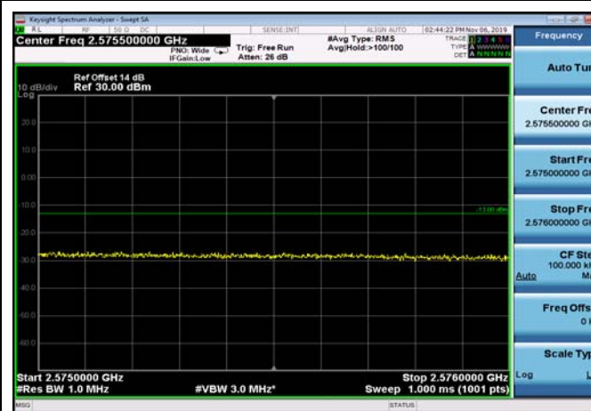
FDD07_10MHz_2565_QPSK_fullIRB_ExtraBan ds_Range_2575~2576
