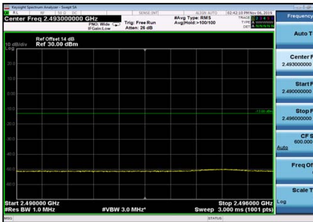
FDD07_10MHz_2565_QPSK_OneRB_low _ExtraBands_Range_2490~2496
