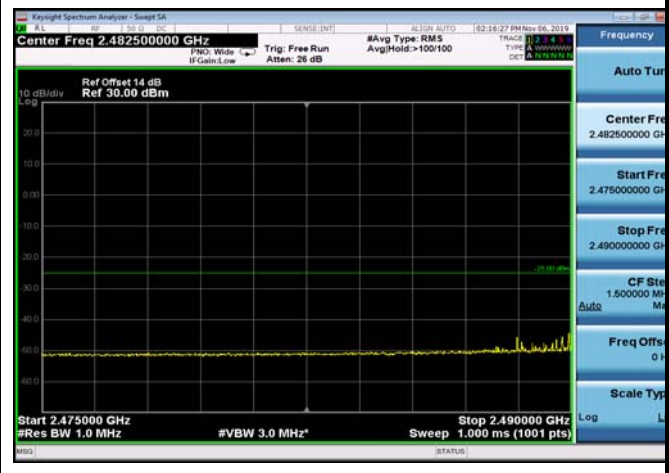
FDD07_5MHz_2502.5_Q16_OneRB_low _ExtraBands_Range_2475~2490
