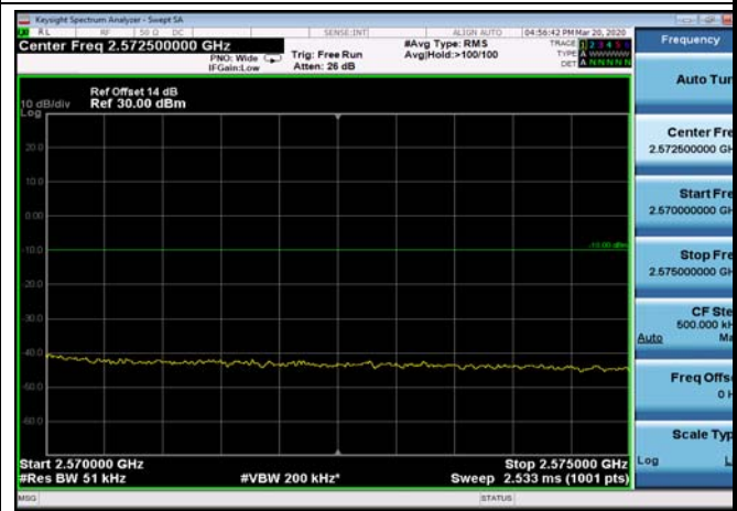
FDD07_20MHz_2560_QPSK_fullIRB_ExtraBan ds_Range_2570~2575
