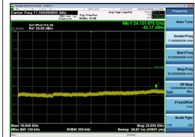
,Plot 5,10000MHz~25000MHz-802.11n(HT40),2452MHz,Ant0
