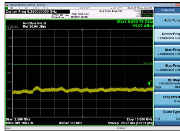
,Plot 4,2500MHz~10000MHz-802.11n(HT40),2452MHz,Ant0
