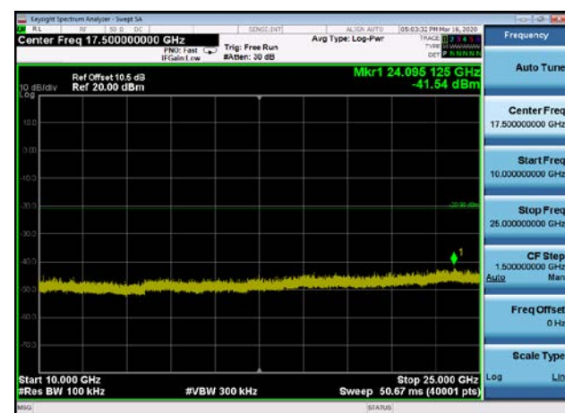
,Plot 5,10000MHz~25000MHz-802.11n(HT40),2437MHz,Ant0
