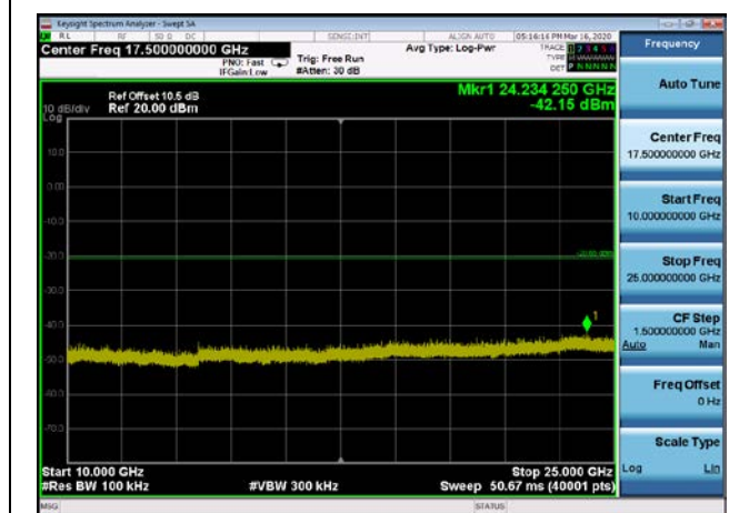
,Plot 5,10000MHz~25000MHz-802.11n(HT40),2452MHz,Ant0
