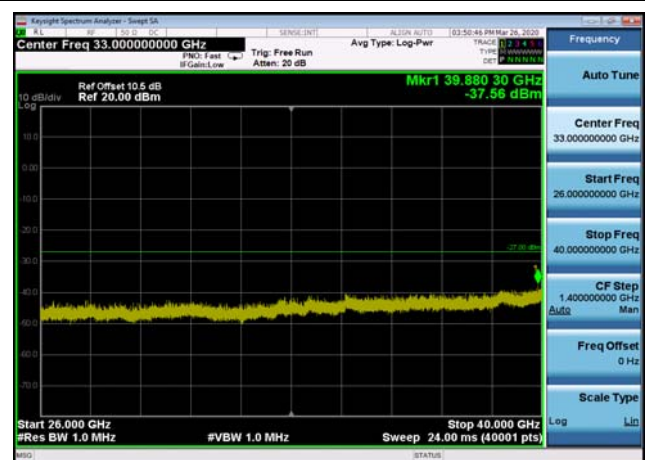
U-NII-1 ,Plot 4,26000MHz~40000MHz-802 .11n(40MHz),5230MHz,Ant1
