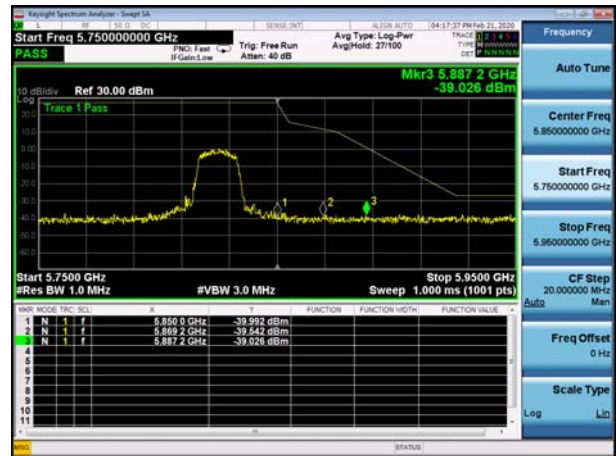
U-NII-3 Band Edge-802.11ac(20MHz) ,5825MHz
