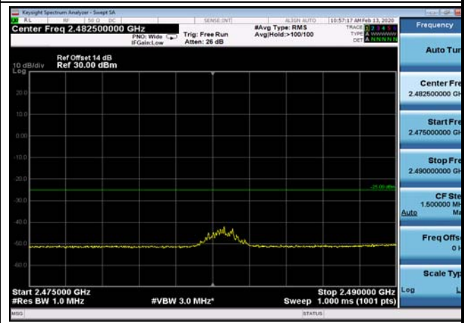
FDD07_10MHz_2505_Q16_OneRB_low _ExtraBands_Range_2475~2490
