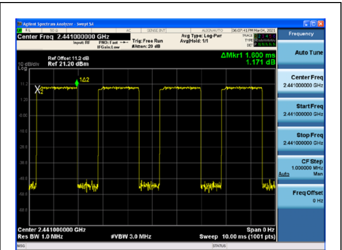
Modulation: \pi/4 DQPSK DH3 2441
