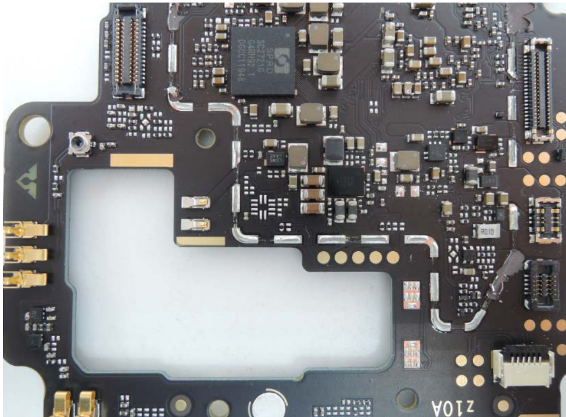
IC Details 11
