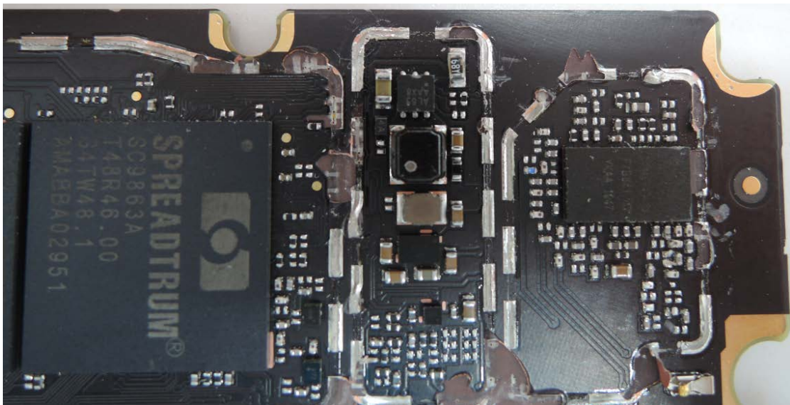
IC Details 6
