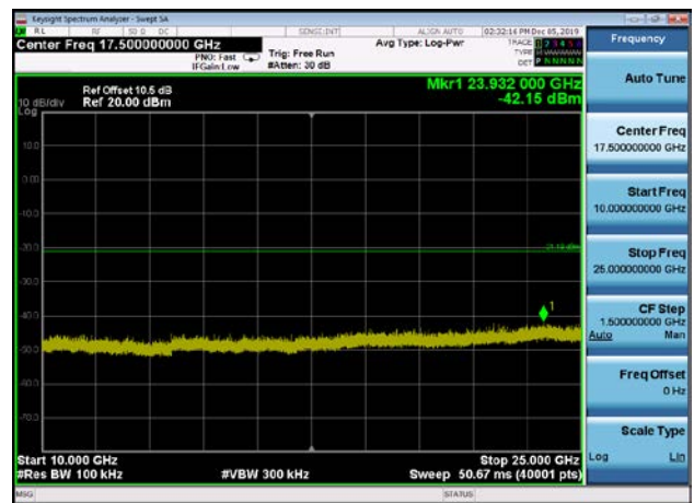
,Plot 5,10000MHz~25000MHz-802.11n(HT40),2452MHz
