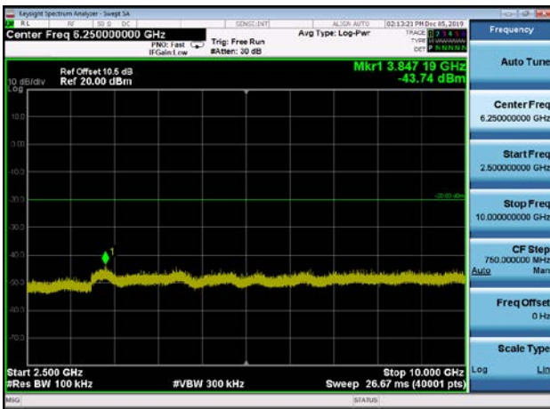
,Plot 4,2500MHz~10000MHz-802.11n(HT40),2452MHz
