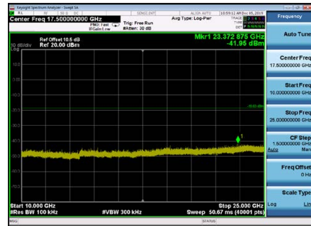
,Plot 5,10000MHz~25000MHz-802.11n(HT20),2462MHz
