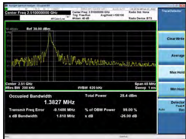
DC_28A (Subset 1)-n7A 64QAM 1RB 20MHz CH-Middle
