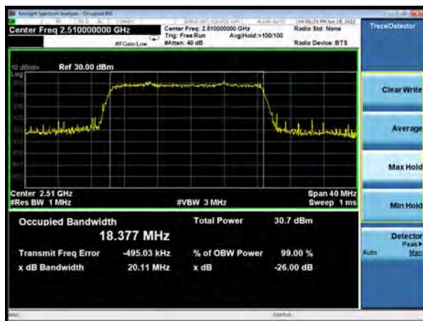
DC_28A (Subset 1)-n7A QPSK 100%RB 20MHz CH-Middle
