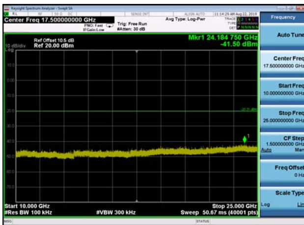
,Plot 5,10000MHz~25000MHz-802.11n(HT40),2437MHz,Ant0
