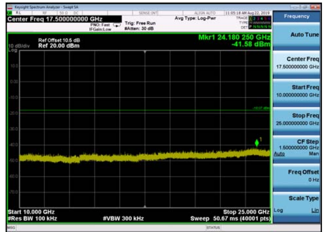
,Plot 5,10000MHz~25000MHz-802.11n(HT40),2452MHz,Ant0
