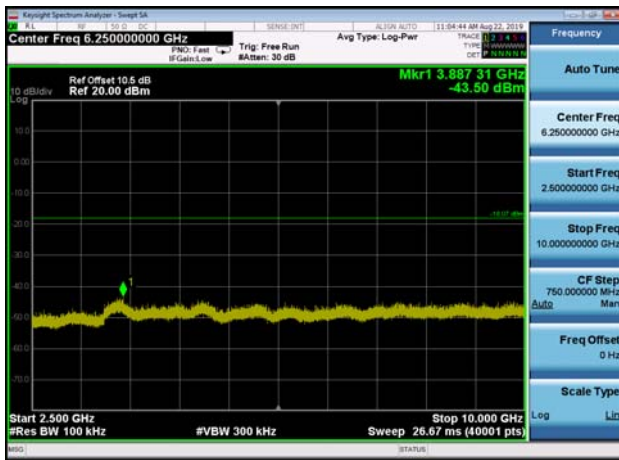
,Plot 4,2500MHz~10000MHz-802.11n(HT40),2452MHz,Ant0
