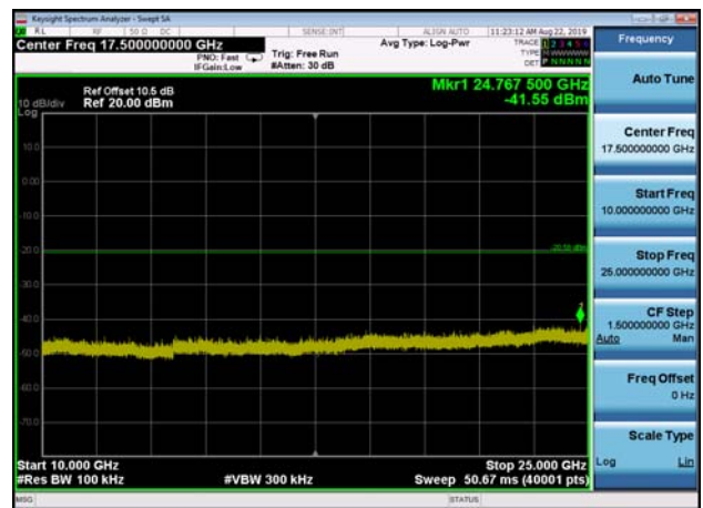
,Plot 5,10000MHz~25000MHz-802.11n(HT40),2452MHz,Ant0
