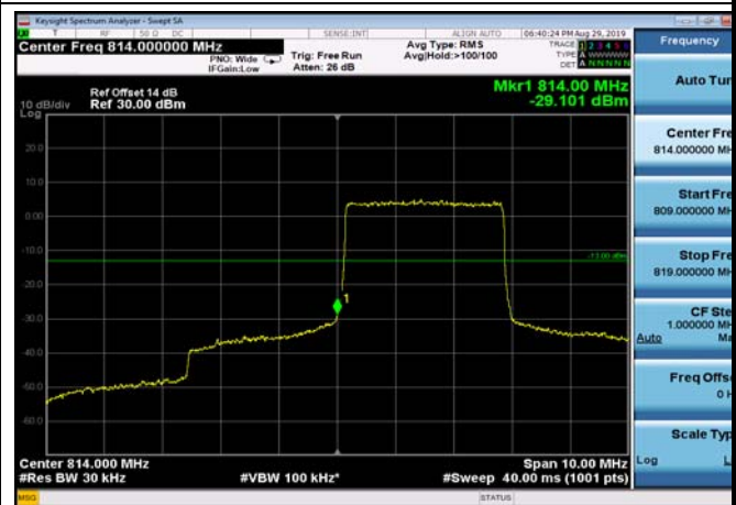
LowRange_FDD26_5MHz_816.5_OneRB_low_Q16
