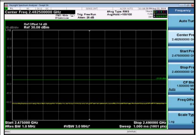
FDD07_5MHz_2567.5_QPSK_OneRB_low _ExtraBands_Range_2475~2490
