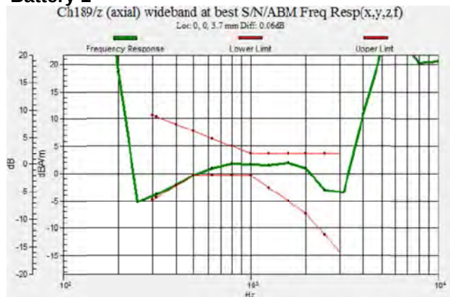
Fig 7.1 GSM850 Ch189
