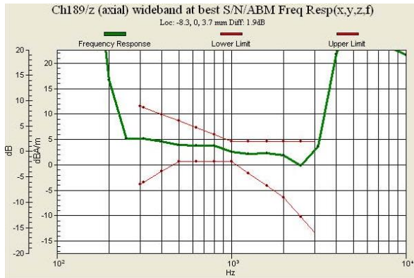
Fig 7.1 GSM850 Ch189
