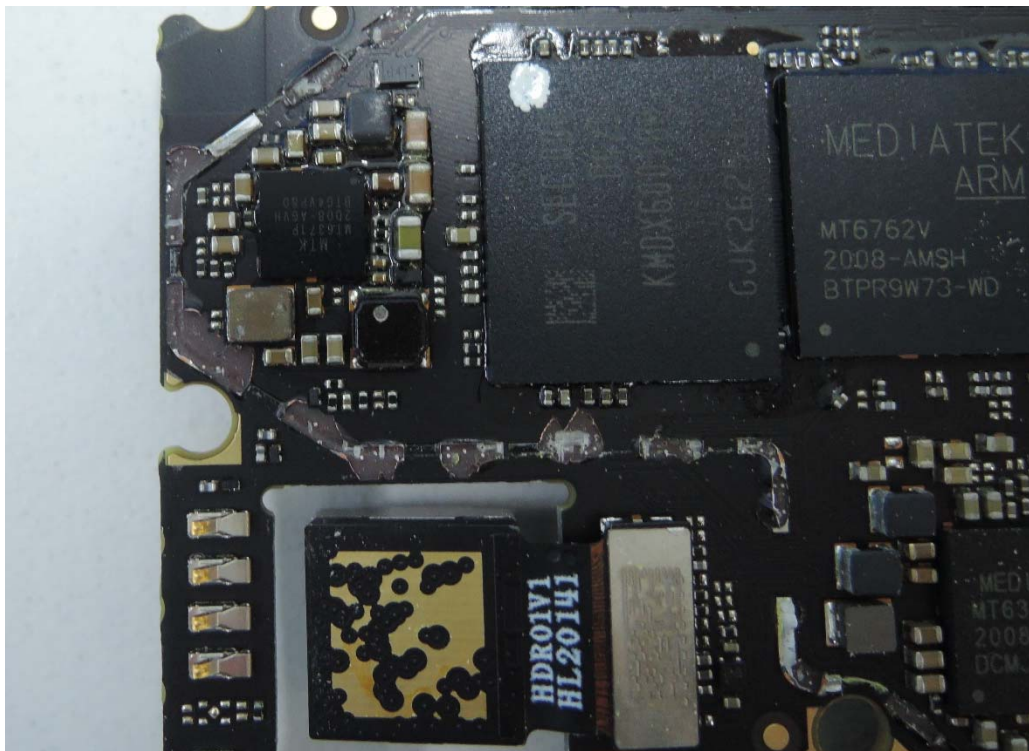
IC Details 8
