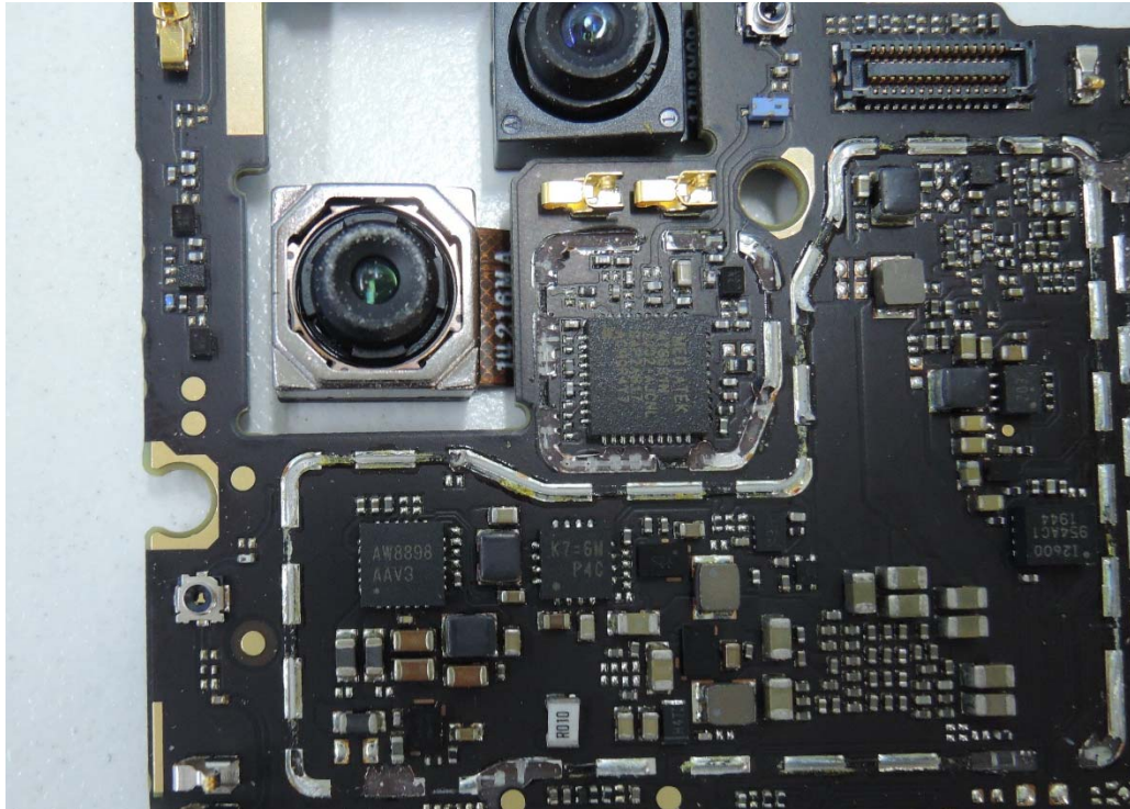
IC Details 3
