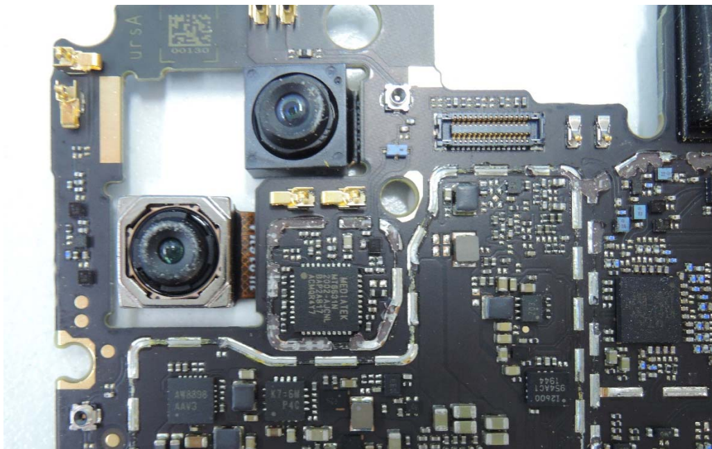
IC Details 2
