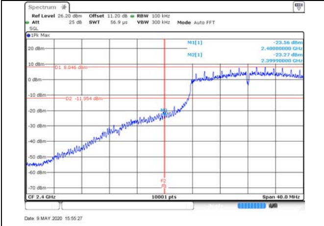
802.11n (HT20)
