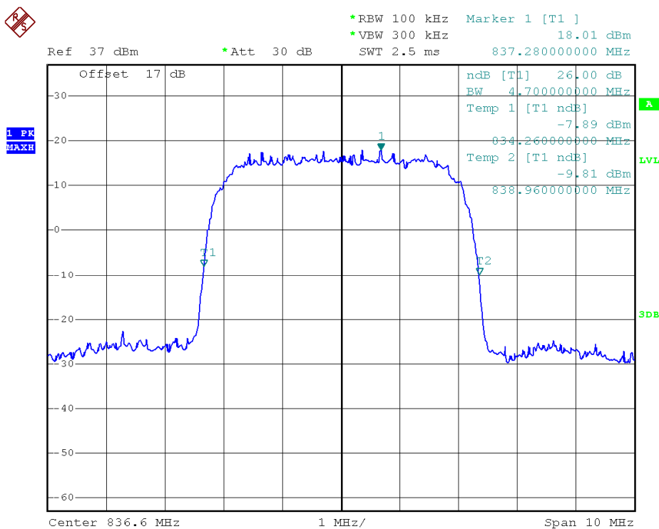
(Plot E2: WCDMA 850MHz Channel = 4183)
