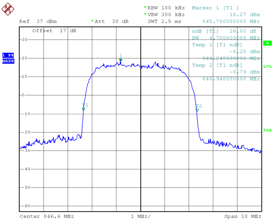
(Plot E3: WCDMA 850MHz Channel = 4233)
