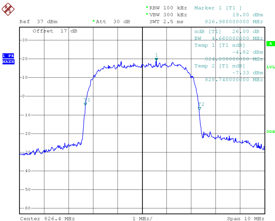
(Plot E1: WCDMA 850MHz Channel = 4132)
