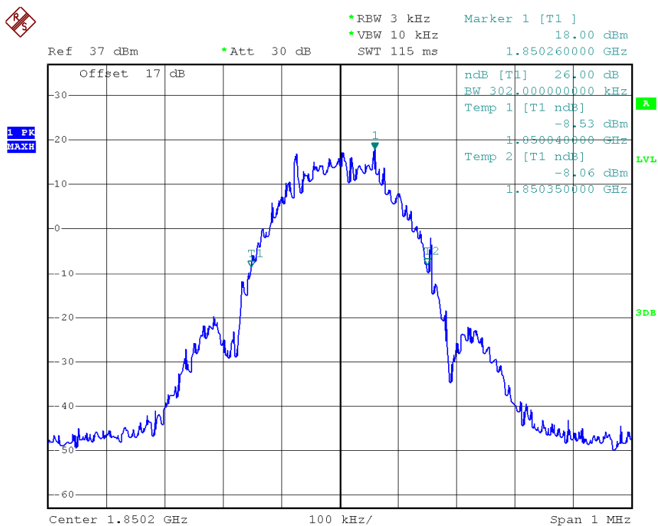
(Plot D1: EDGE 1900MHz Channel = 512)
