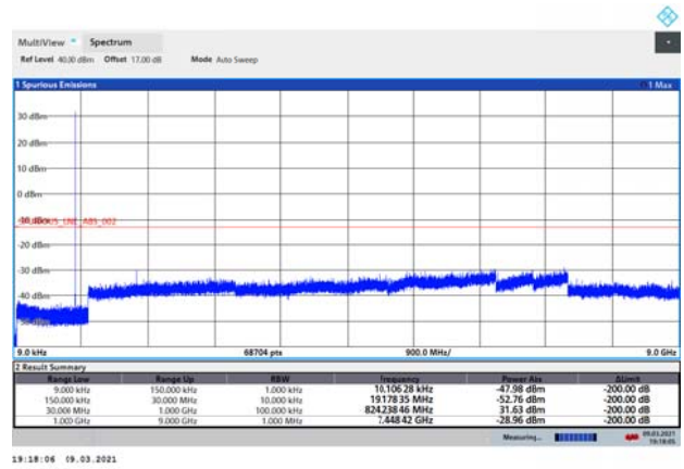
GPRS 850 CH-Middle 9kHz ~ 9GHz
