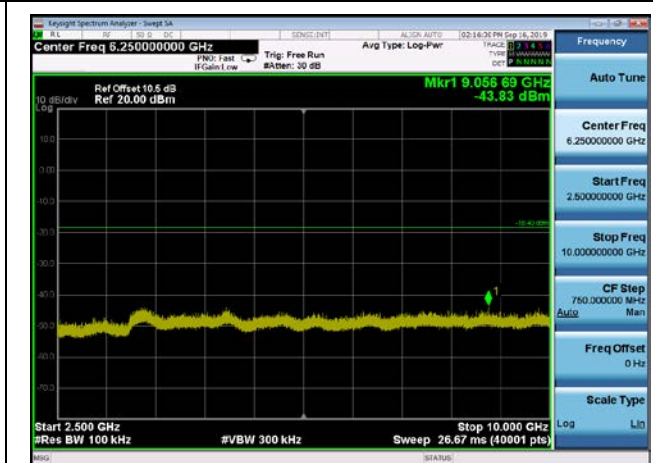
,Plot 4,2500MHz~10000MHz-802.11n(HT20),2462MHz,Ant1
