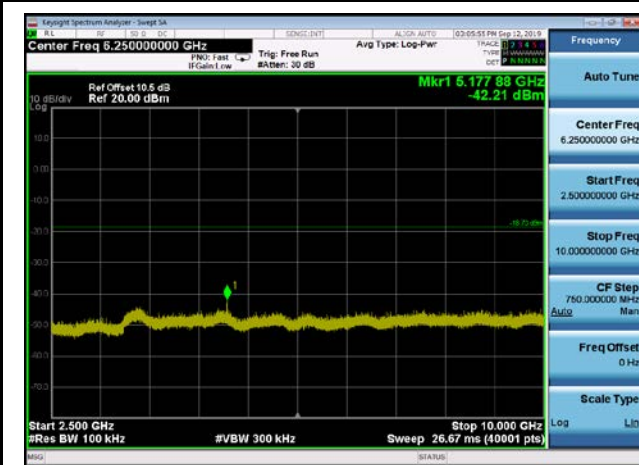
,Plot 4,2500MHz~10000MHz-802.11n(HT20),2437MHz,Ant0
