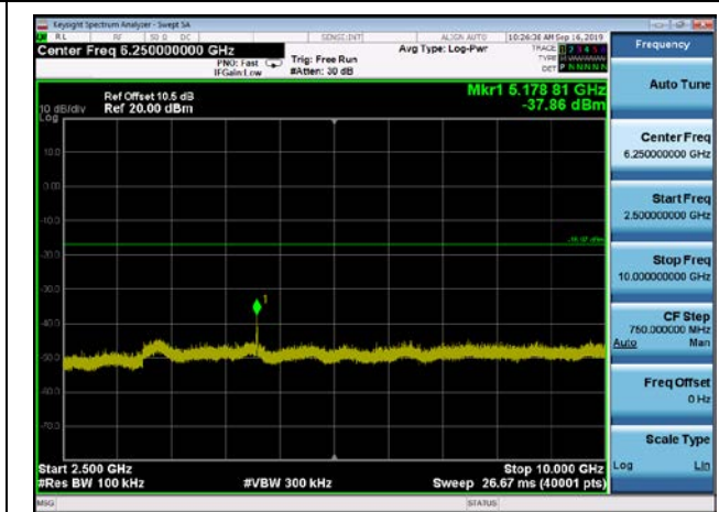
,Plot 4,2500MHz~10000MHz-802.11n(HT20),2437MHz,Ant1
