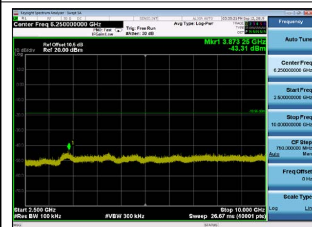
,Plot 4,2500MHz~10000MHz-802.11n(HT20),2462MHz,Ant0
