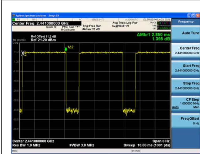
Modulation: \pi/4 DQPSK DH5 2441
