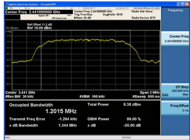
Modulation: \pi/4 DQPSK 2441MHz
