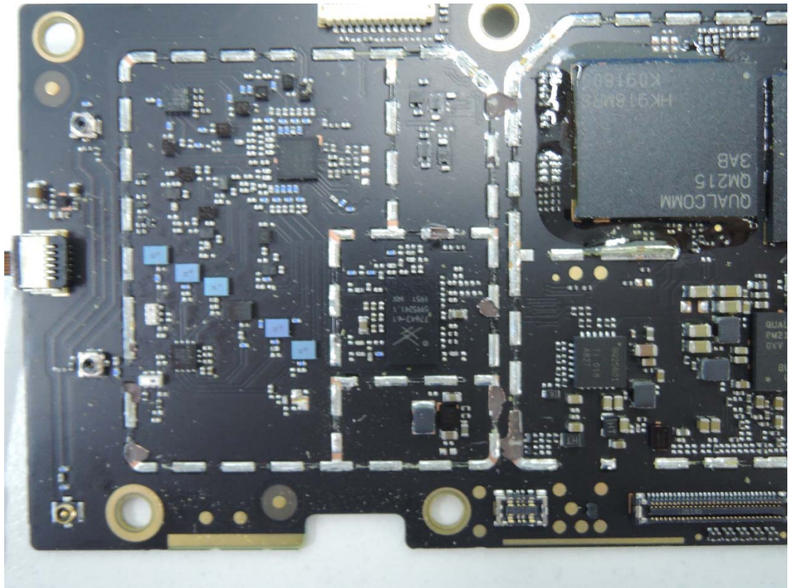
IC Details 3
