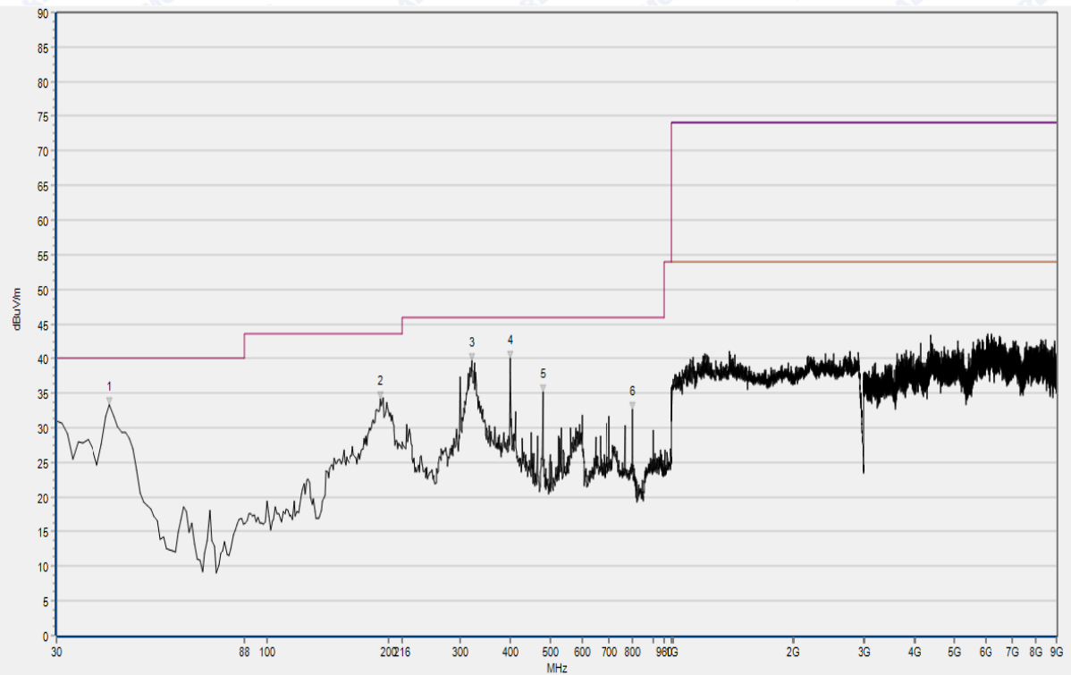
(Plot A: 30MHz – 9GHz, Test Antenna Vertical)
